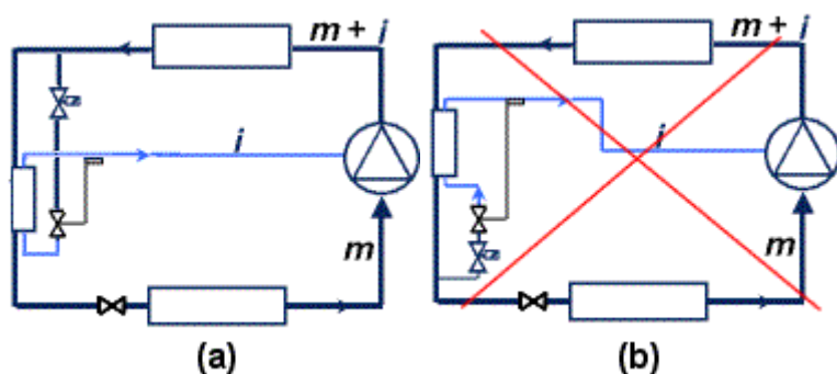
Рис. 9: (а) отбор жидкости выше по течению (рекомендуется) – (b) ниже по течению (не рекомендуется)
